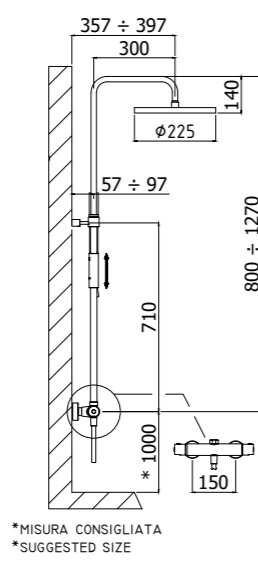
ZCOL 646LIQCR BIRILLO Colonna doccia con miscelatore termostatico Shower column with thermostatic mixer
