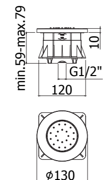
ZSOF 120CR Soffione tondo in ABS, anticalcare, con getto orientabile - Ø130 mm Round ABS body jet, antiscaling system, with swivelling spray - Ø130 mm
