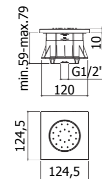
ZSOF 121CR Soffione quadro in ABS, anticalcare, con getto orientabile - 124,5x124,5 mm Square ABS body jet, antiscaling system, with swivelling spray - 124,5x124,5 mm
