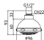
ZSOF 030CR ISCHIA Soffione "Ischia" in ABS, anticalcare Ø 96 mm "Ischia" ABS shower head, antiscald system Ø 96 mm
