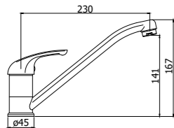
APM 182CR Miscelatore lavello monoforo con canna tubo orientabile One-hole sink mixer with tube swivelling spout
