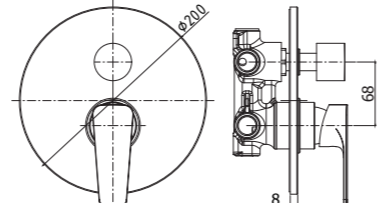
SY 018-019CR Miscelatore incasso doccia con deviatore 2 uscite /3 uscite Concealed shower mixer with diverter 2 outlets /3 outlets
