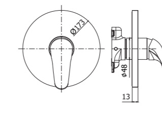
DU BOX010CR Set esterno miscelatore incasso doccia senza deviatore External set for concealed shower mixer without diverter
