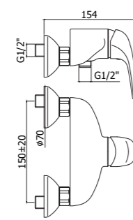
DU 168-168DCR Miscelatore doccia con/senza set doccia Shower mixer with/without shower set
