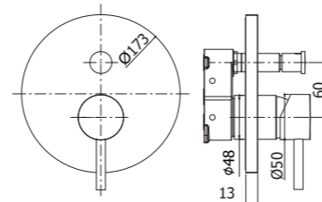
BI BOX015CR Set esterno miscelatore incasso doccia con deviatore External set for concealed shower mixer with diverter
