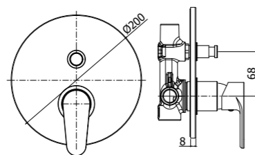
GR 015CR Miscelatore incasso doccia con deviatore Concealed shower mixer with diverter
