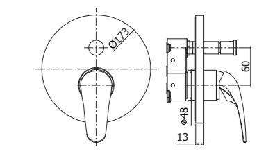
DU BOX015CR Set esterno miscelatore incasso doccia con deviatore External set for concealed shower mixer with diverter
