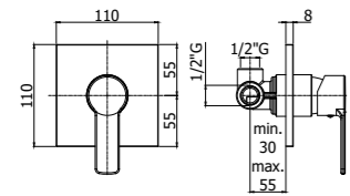
RED 010CR Miscelatore incasso doccia Concealed shower mixer
