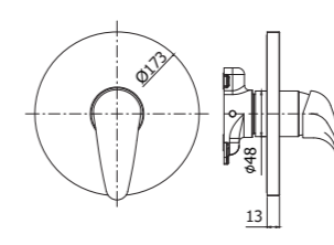
ND BOX010CR Set esterno miscelatore incasso doccia senza deviatore External set for concealed shower mixer without diverter
