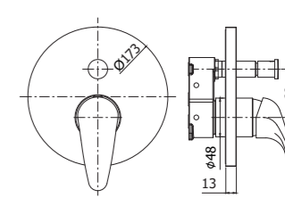
ND BOX015CR Set esterno miscelatore incasso doccia con deviatore External set for concealed shower mixer with diverter
