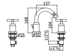
QTV 119-118CR Batteria bidet con bocca erogazione, con/ senza scarico Three-hole bidet mixer with spout, with/ without pop up waste
