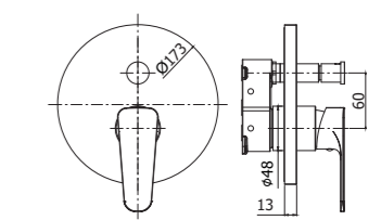
SY BOX015CR Set esterno miscelatore incasso doccia con deviatore External set for concealed shower mixer with diverter
