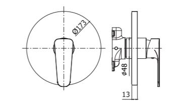
SY BOX010CR Set esterno miscelatore incasso doccia senza deviatore External set for concealed shower mixer without diverter
